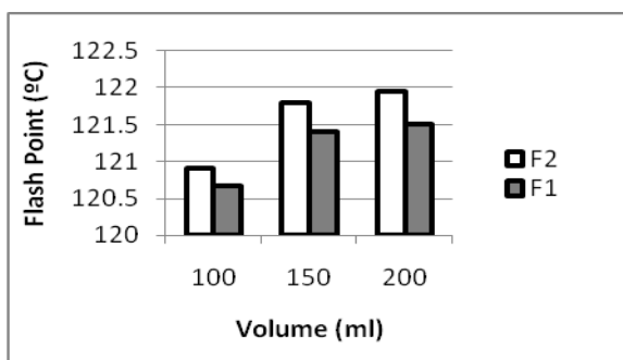
Gambar 9. Flash Point biodiesel minyak jarak pagar pada berbagai perbandingan co-solvent dan Volume
