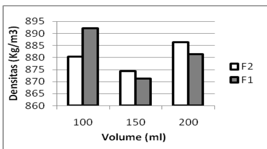
Gambar 7. Densitas biodiesel minyak jarak pagar pada berbagai perbandingan co-solvent dan Volume
