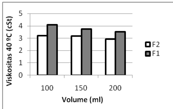
Gambar 8. Viskositas biodiesel minyak jarak pagar pada berbagai perbandingan co-solvent dan Volume
