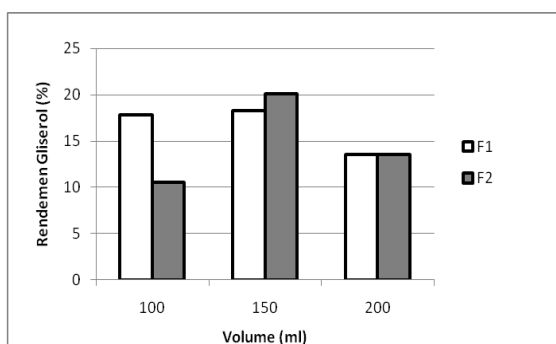
Gambar 6. Rendemen biodiesel minyak jarak pagar pada berbagai perbandingan co-solvent dan Volume
