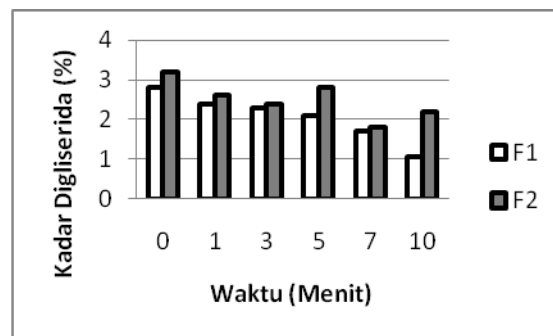
Gambar 4. Kandungan Digliserida biodiesel minyak jarak pagar pada berbagai perbandingan co-solvent dan lama pengambilan
