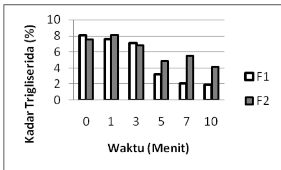
Gambar 3. Kandungan Trigliserida biodiesel minyak jarak pagar pada berbagai perbandingan co-solvent dan lama pengambilan
