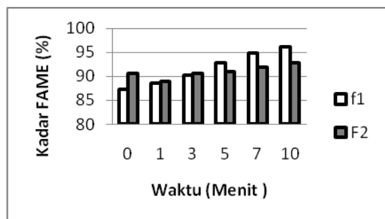
Gambar 2. Kandungan FAME biodiesel minyak jarak pagar pada berbagai perbandingan co-solvent dan lama pengambilan
