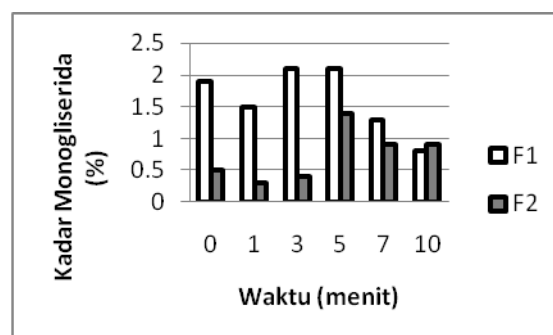
Gambar 5. Kandungan Monogliserida biodiesel minyak jarak pagar pada berbagai perbandingan co-solvent dan lama pengambilan
