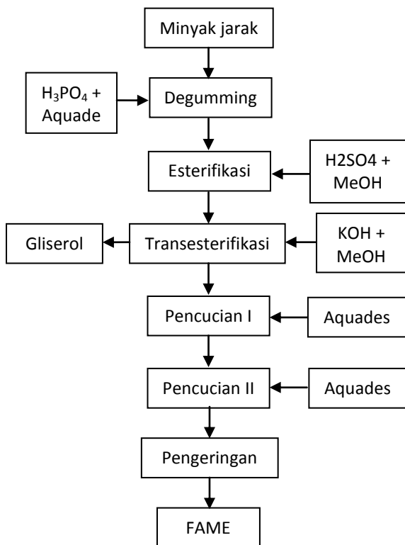
Gambar 1. Langkah-langkah pembuatan biodiesel minyak jarak pagar.
