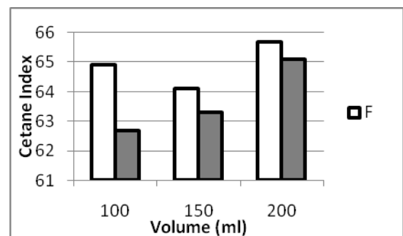
Gambar 10. Cetane Index biodiesel minyak jarak pagar pada berbagai perbandingan co-solvent dan Volume
